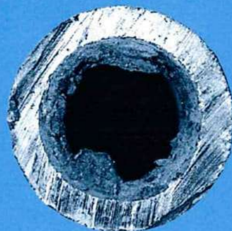
鉄サビや汚れが付着した水道管の断面写真(一例)
